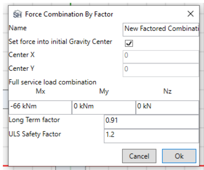
Рисунок 4-32. Ввод данных по загрузению
