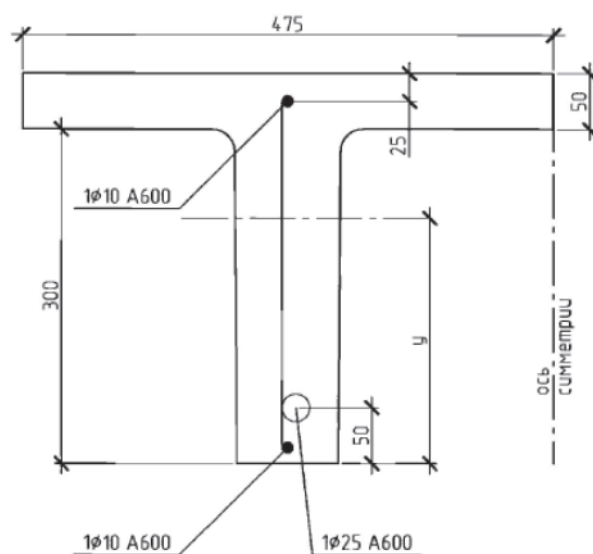
Рисунок 4-28. Поперечное сечение ребристой плиты по данным источника Ввод исходных данных в StructureHelper
