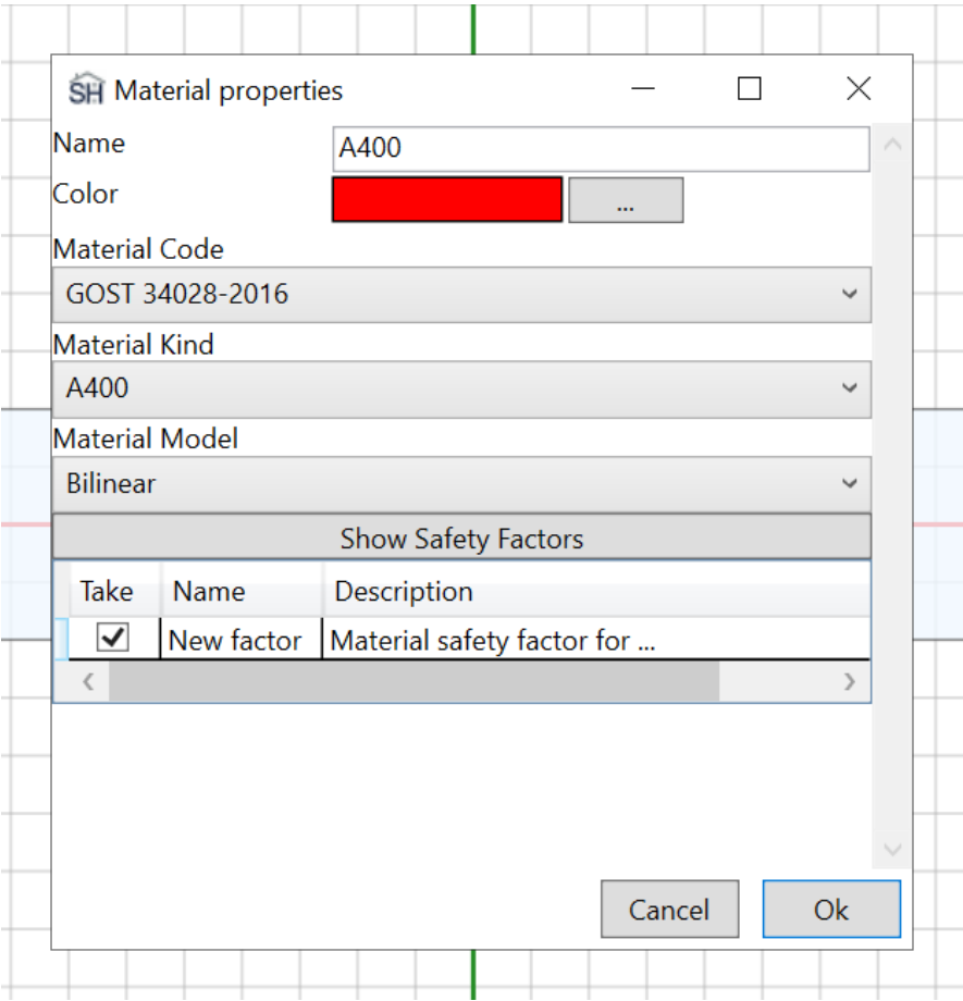
Рисунок 4-25. Свойства материала для арматуры
