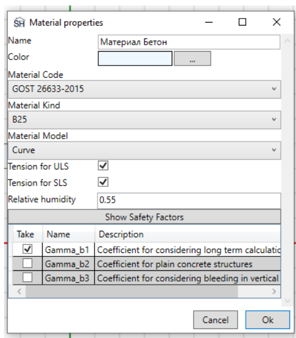
Рисунок 4-30. Материал бетона
