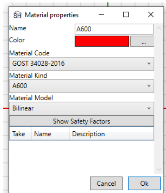
Рисунок 3-55. Материал арматуры.
