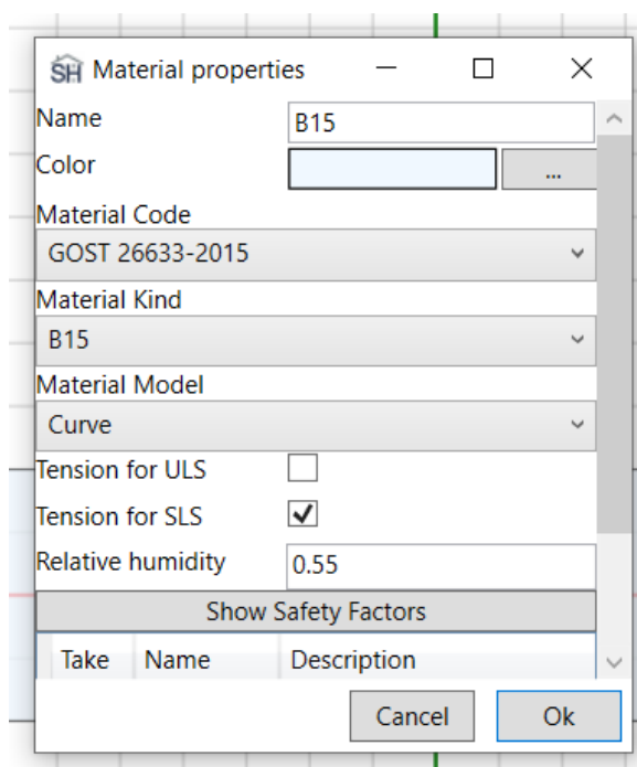
Рисунок 4-24. Свойства материала для бетона
